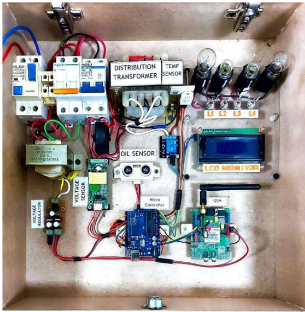
Fig.6FinalPrototype
